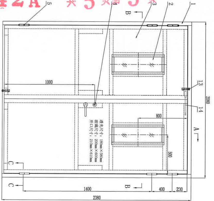
背面立面图
