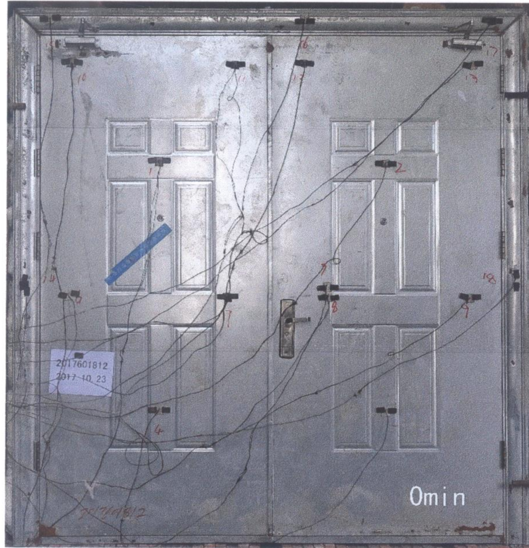
照片 1 耐火试验前试件情况
