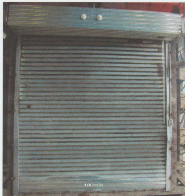
照片 2 耐火试验结束时试件情况
