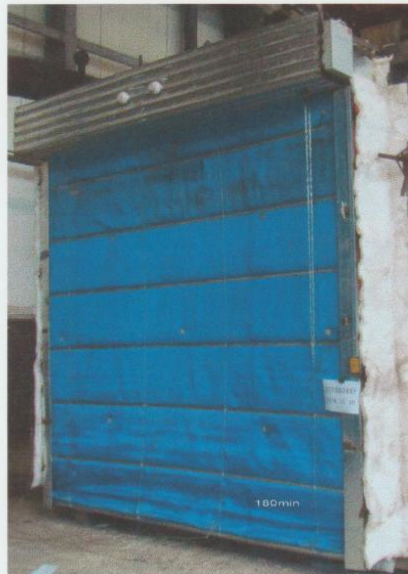
照片 2 耐火试验结束时试件情况
